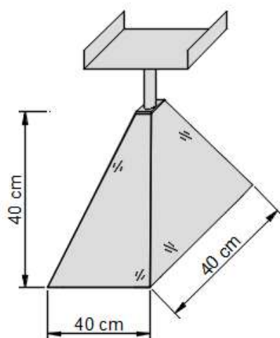
Figura 7. Base aislada transportable.
