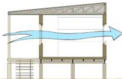
Figura 6. Funcionamiento vivienda unifamiliar y piezas partes de paneles.
