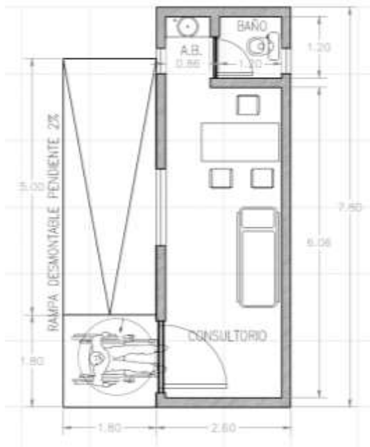
Figura 2. Módulo, sala primeros auxilios.
