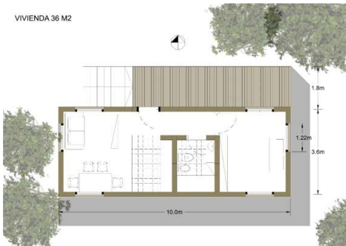
Figura 4. Modulo vivienda, planta.
